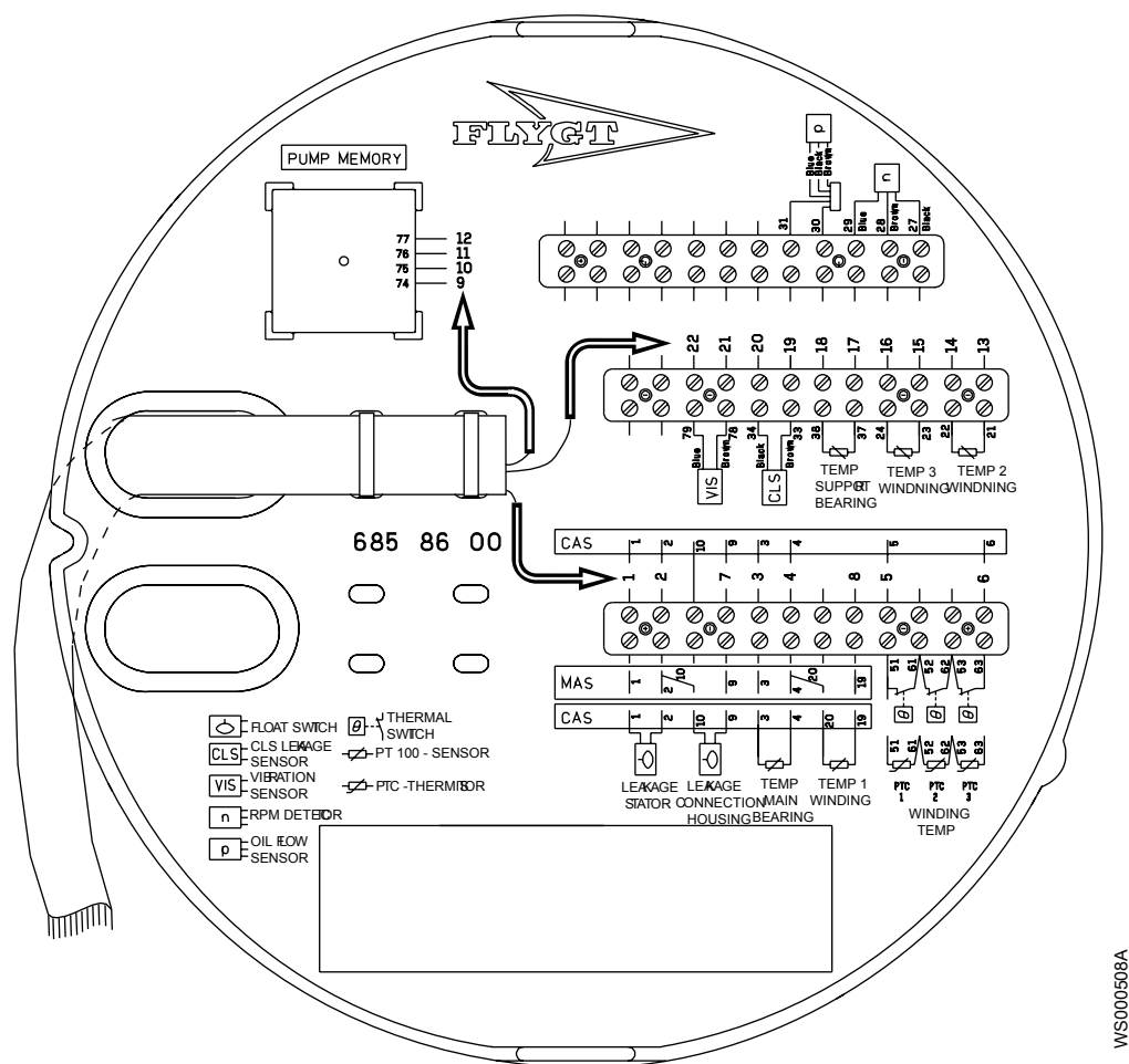
Рис. 22: Подключения устройства. Стрелки указывают номера проводов кабеля SUBCAB
