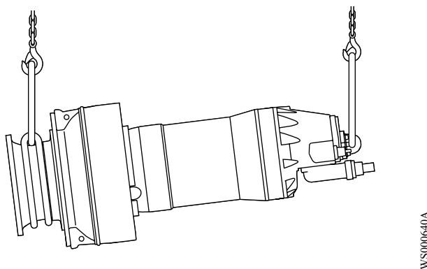
Рис. 35: Поднимите агрегат для ремонта. Показан типовой насос.
