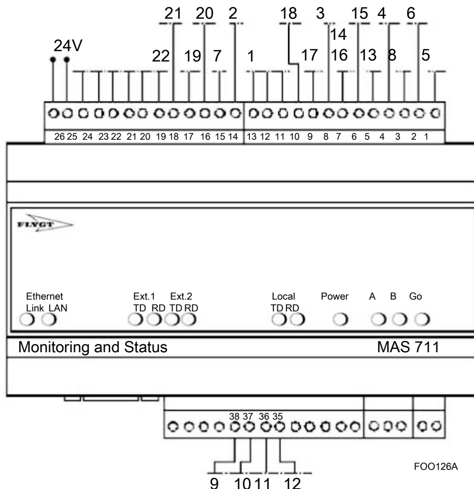
Рис. 23: Подключения к основному блоку MAS 711.
