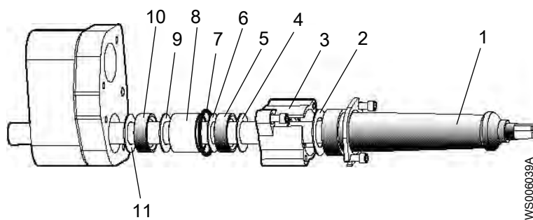
Рис. 16: Блоки привода 605-776
