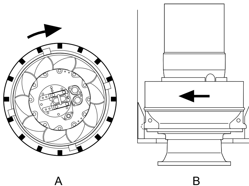
Рис. 33: Вид сверху (А) и вид сбоку (В)
