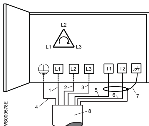
Рис. 27: Правильное чередование фаз
