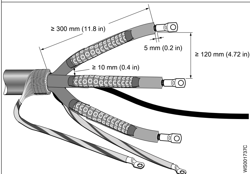
Рис. 29: Рекомендуемые расстояния
